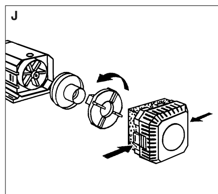
EHEIM universal 1200 / 2400 / 3400 / 4500
