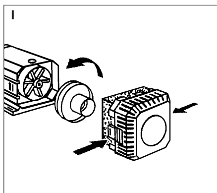
EHEIM universal 300 / 600
