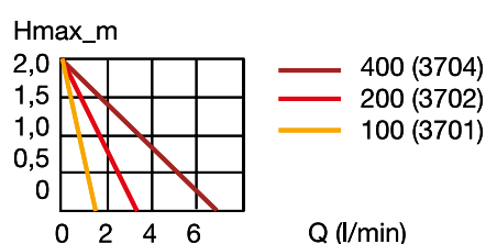
Diagramme de débit des pompes à air
