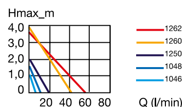
Diagramme de débit des pompes universelles
