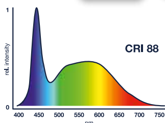
Spectre de couleurs classicLED daylight
