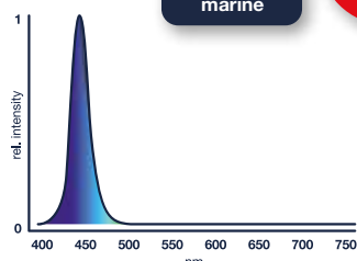
Spectre de couleurs powerLED+ marine actinic
