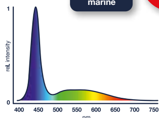
Spéctre de couleurs powerLED+ marine hybrid
