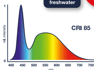
Spectre de couleurs powerLED+ fresh daylight
