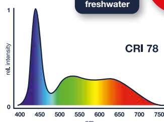
Spectre de couleurs powerLED+ fresh plants
